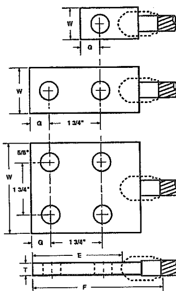
LA Zapata Recta.
