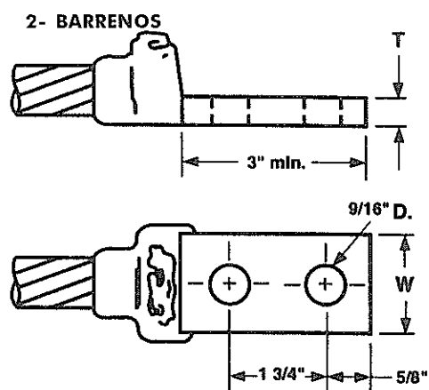
Zapatas Serie -B-122 con barrenado NEMA
